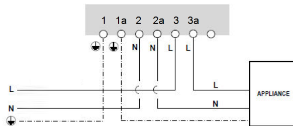
Afbeelding 5: Op het apparaat aansluiten
