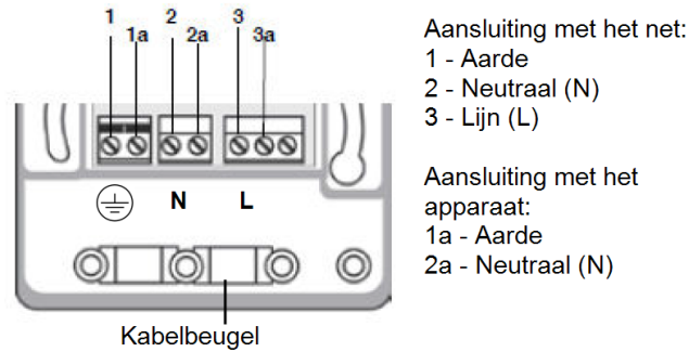
Afbeelding 4: De aansluitingen van de schakelaar met energiemeter
